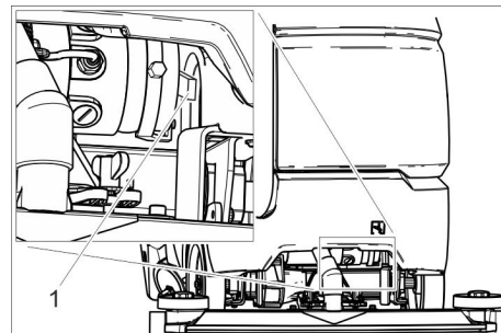
1 Spärrspak
