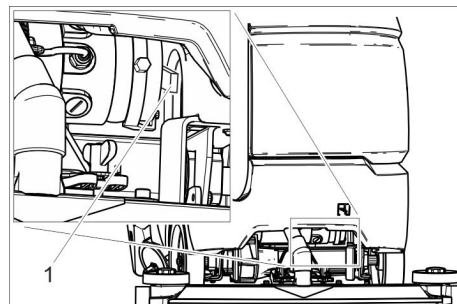
1 Kioldókar
